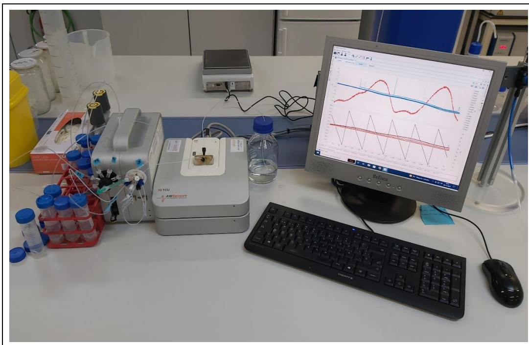
Figura 1. Prototipo de sistema biosensor.
